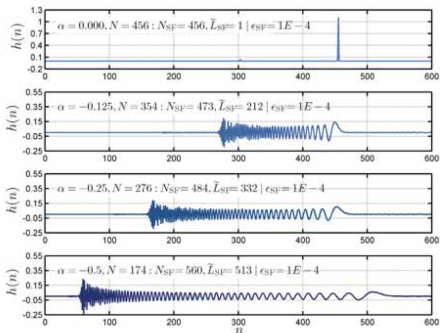
Рис. 5. Импульсные характеристики систем анализ/синтез с различными параметрами N и \alpha
