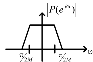
Рис. 6. Типичная АЧХ фильтра-прототипа
