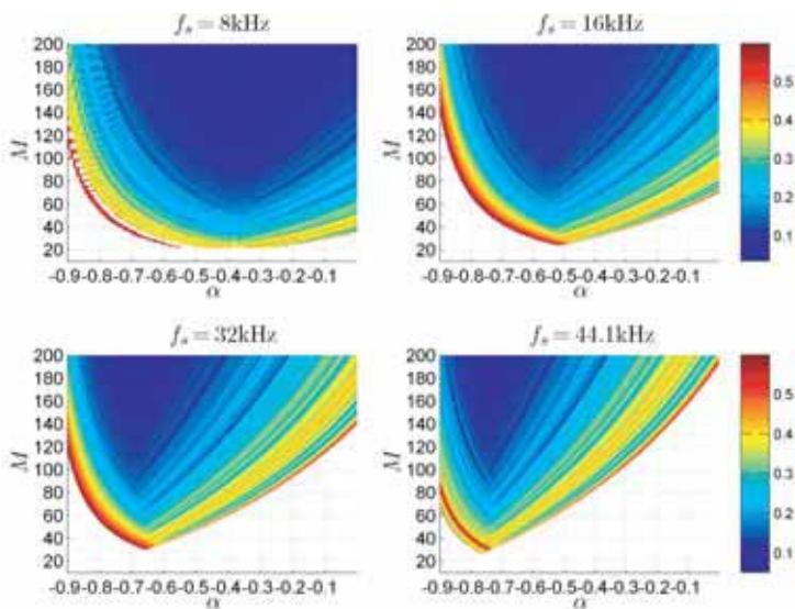
Рис. 7. График профиля максимальной относительной ошибки
