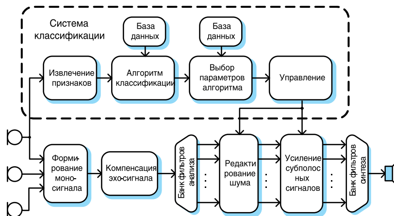
Рис. 1. Стадии обработки сигнала в слуховом аппарате
