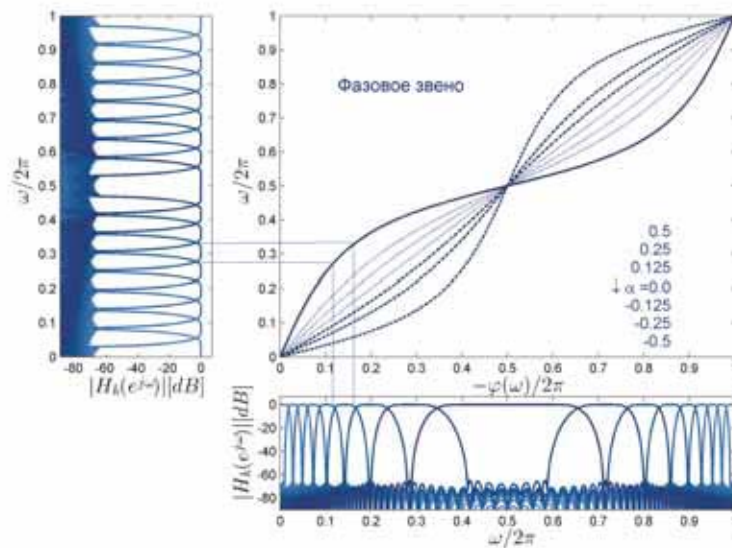
Рис. 2. Фазовое преобразование косинусно-модулированного банка фильтров
