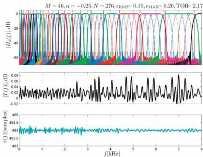
Рис. 9. Частотные характеристики банков фильтров, основанных на деформации оси частот и объединении субполос ( M = 46, N = 276 )
