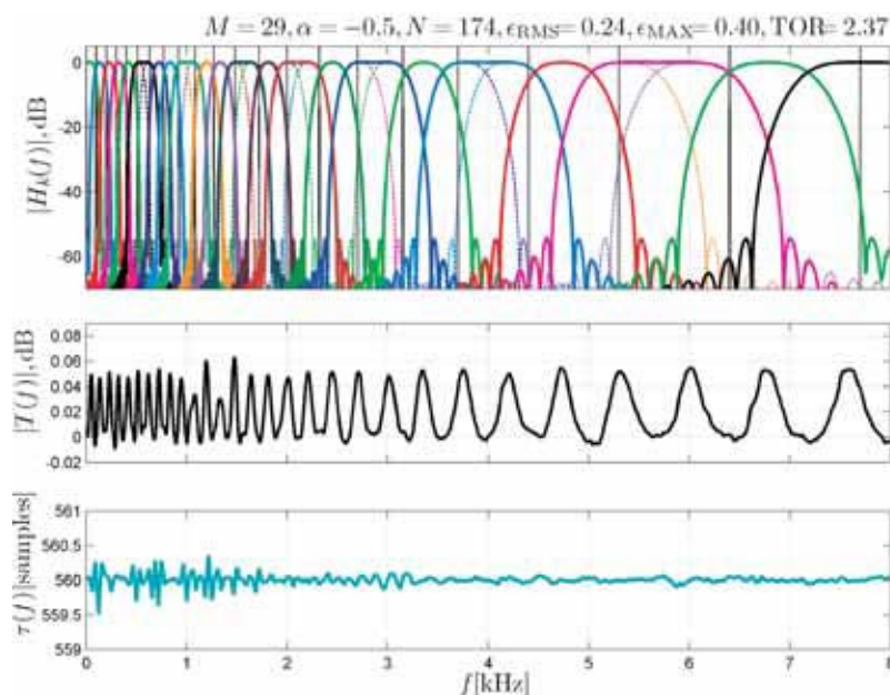
Рис. 8. Частотные характеристики банка фильтров, основанных на деформации оси частот и объединении субполос ( M = 29, N = 174 )
