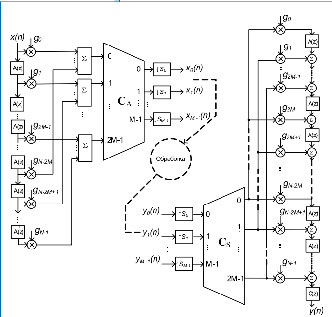
Рис. 3. Структура косинусно-модулированного банка фильтров с деформированной осью частот
