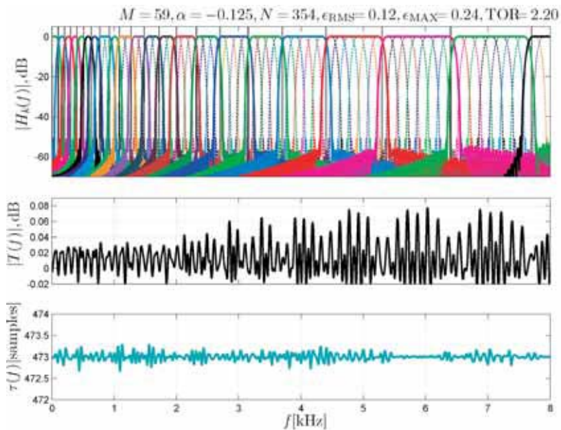
Рис. 10. Частотные характеристики банков фильтров, основанных на деформации оси частот и объединении субполос ( M = 59, N = 354 )
