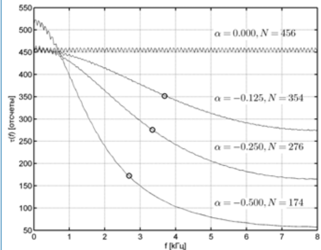
Рис. 4. График групповой задержки для различных банков фильтров
