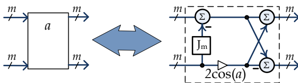
Рис. 2. Базовая операция быстрого алгоритма ДКП-2
