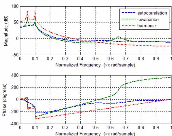
Рис.1. Сравнительный спектральный анализ гармонического сигнала, выполненный различными методами
